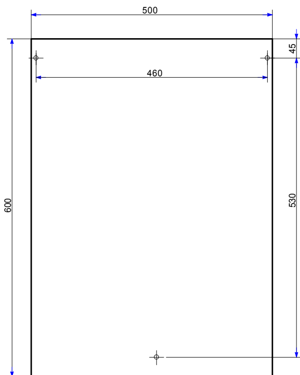
СВТ29.412.000-01(..-08) [1 - 25A]
