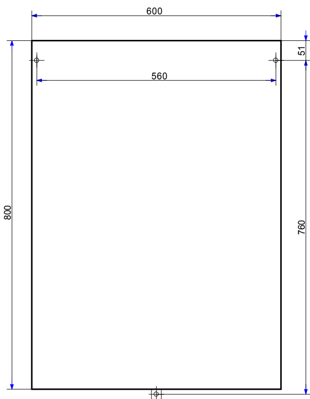
СВТ29.402.000-09(..-13) [32 - 80A]*
