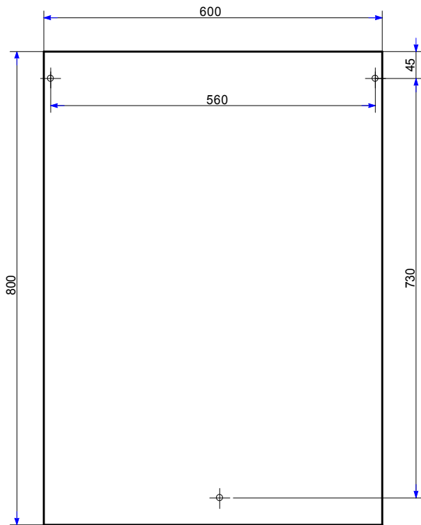
СВТ29.412.000-09(..-13) [32 - 80A]
