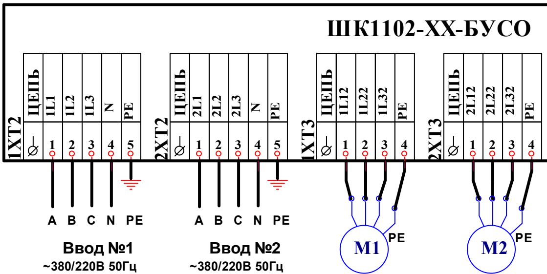
Схема подключения силовых кабелей
