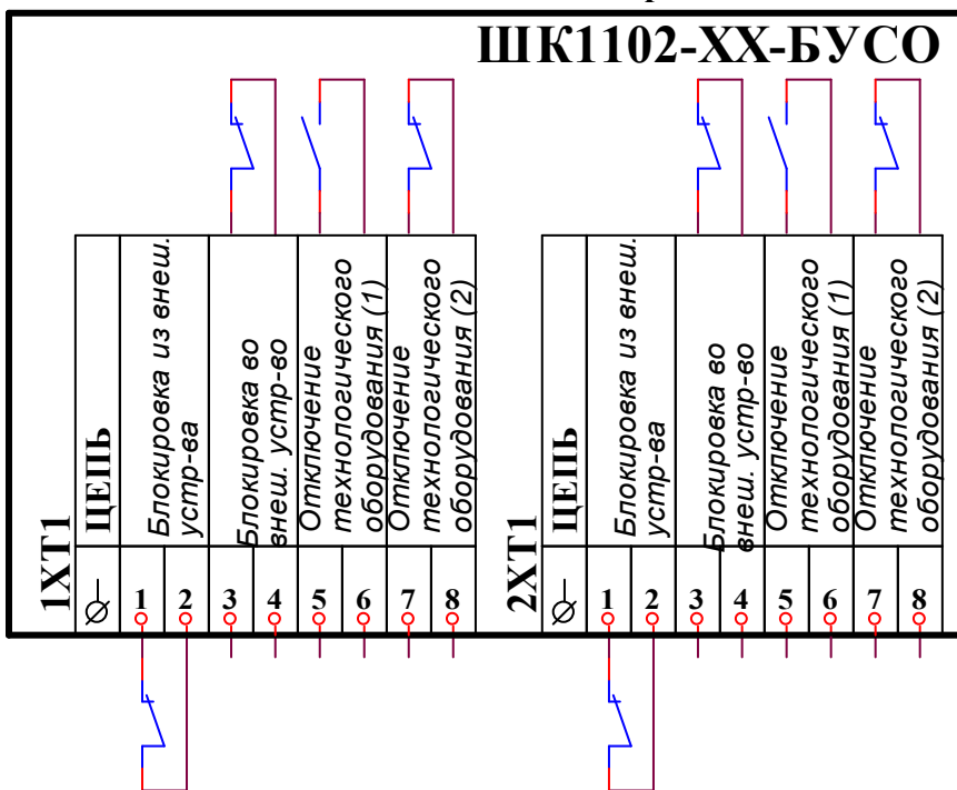
Схема подключения контрольных кабелей
