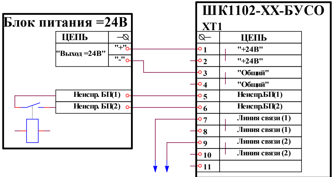
Схема подключения блока питания и линии связи:
